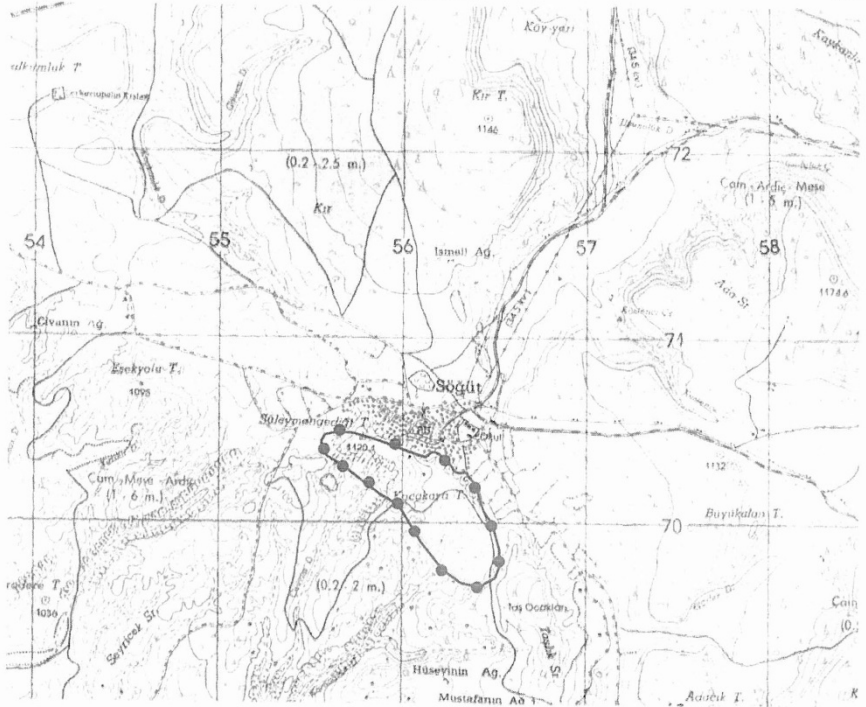
UTM 6 derecelik dilime esas ED50 datumu koordinat değerleri
